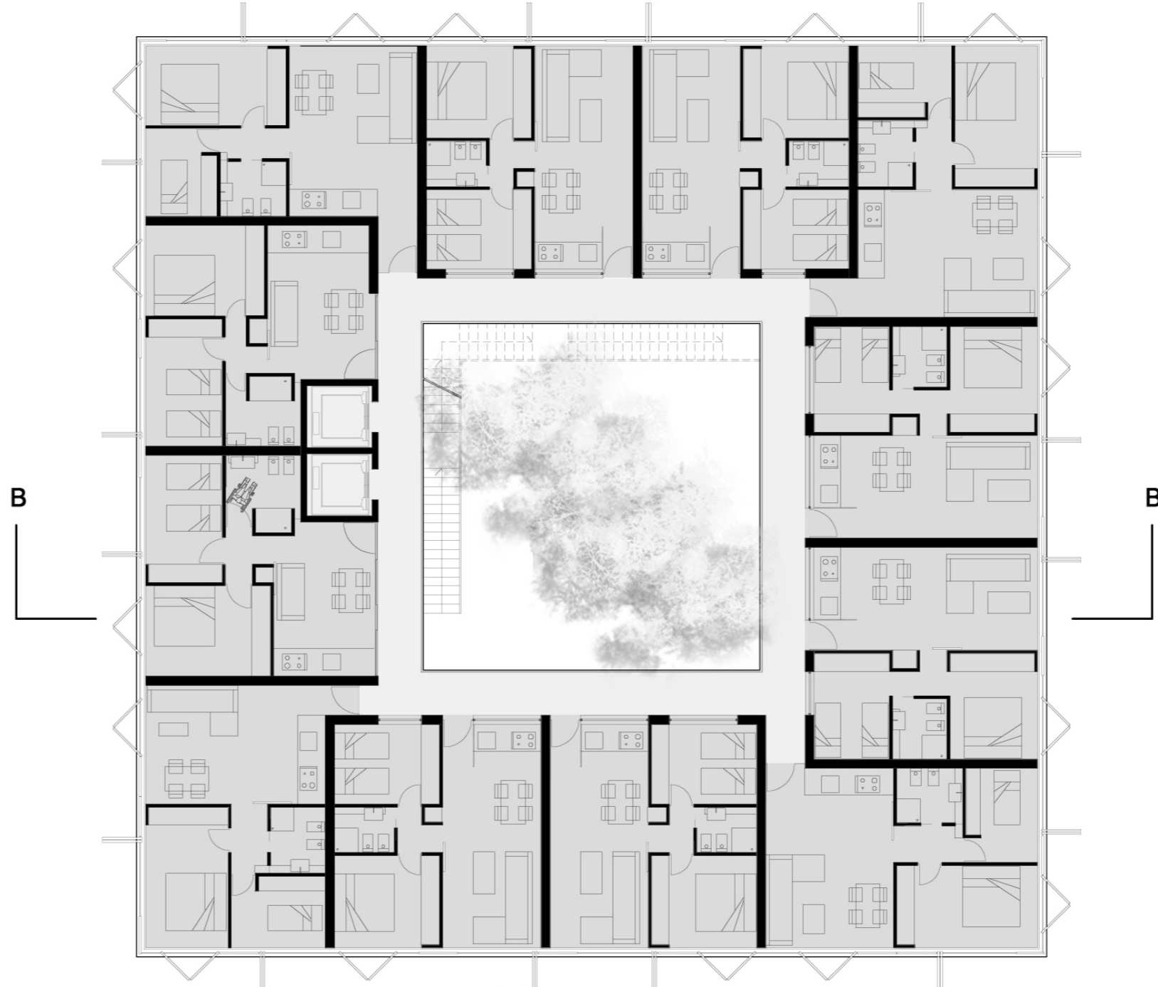
parcela A - planta a escala 1/200
