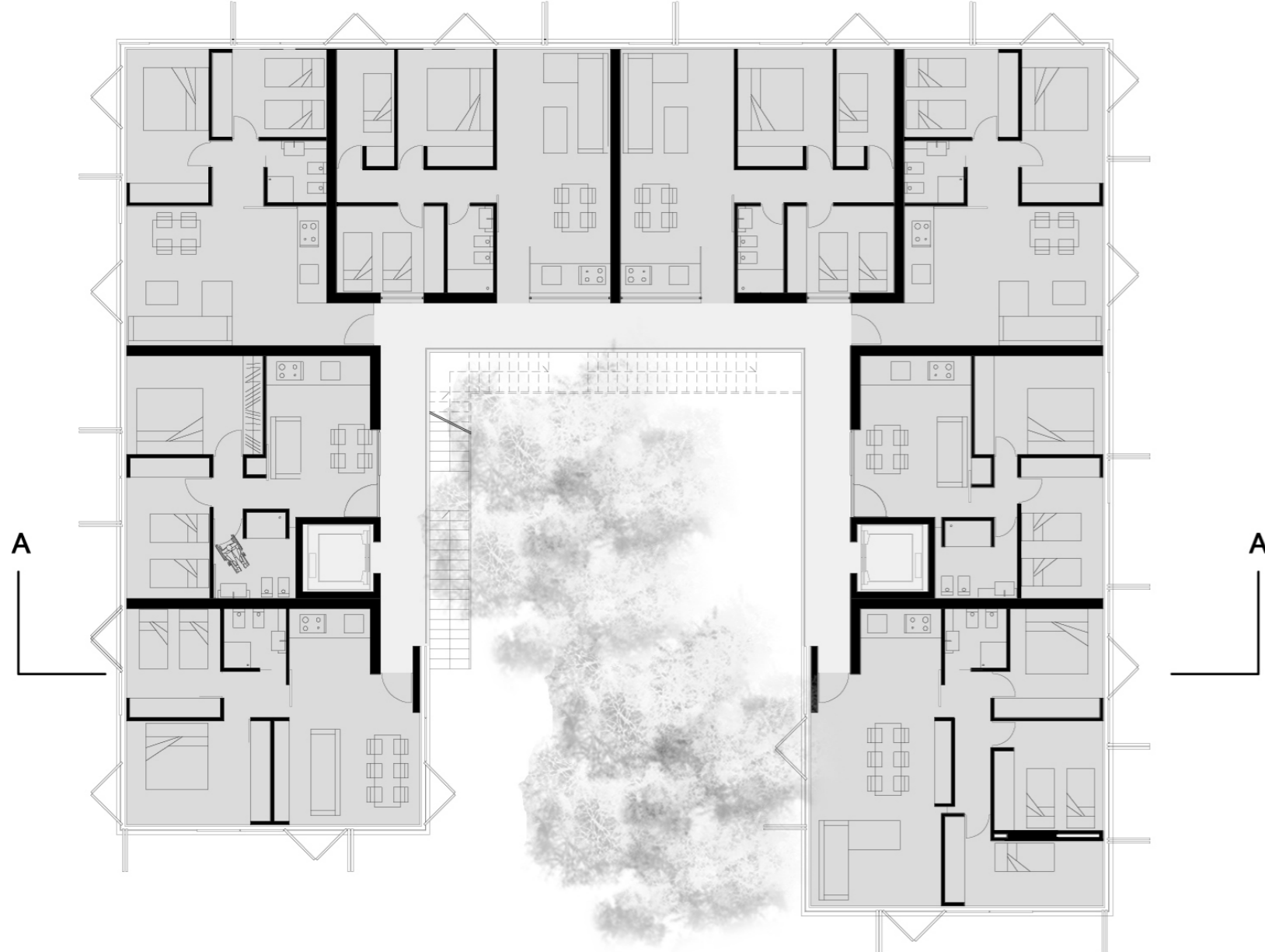
parcela B - planta a escala 1/200
